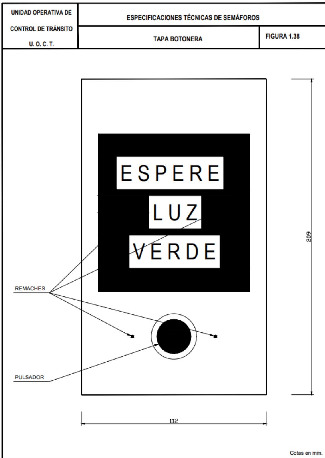
Figura 1.38 Tapa botonera
