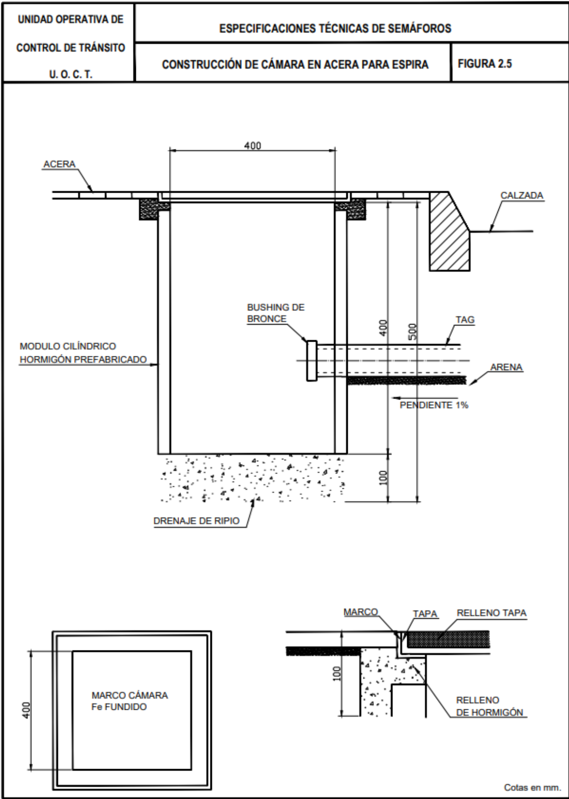
Figura 2.5 Construcción de cámara en acera para espira
