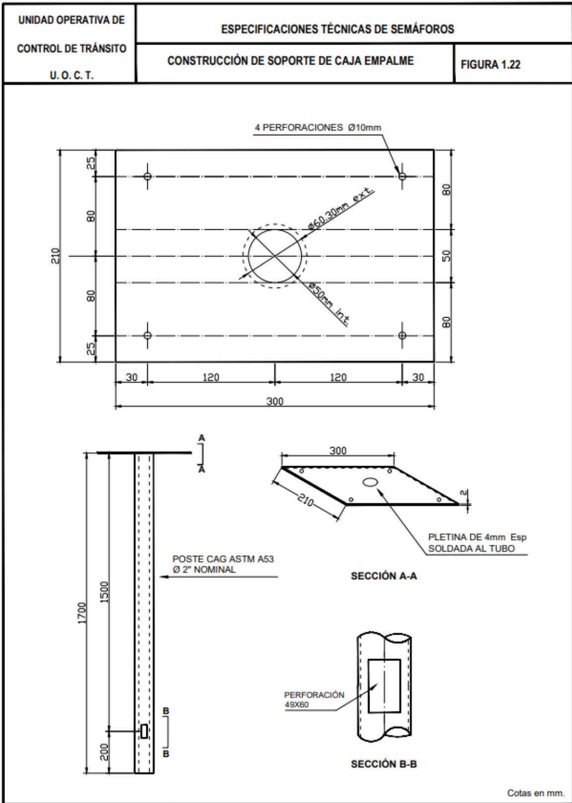
Figura 1.22 Construcción de soporte de caja empalme
