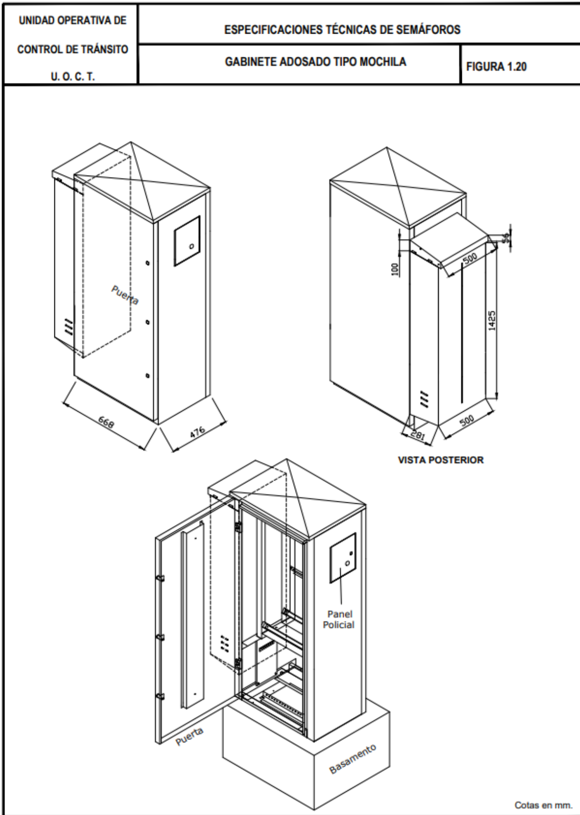
Figura 1.20 Gabinete adosado tipo mochila
