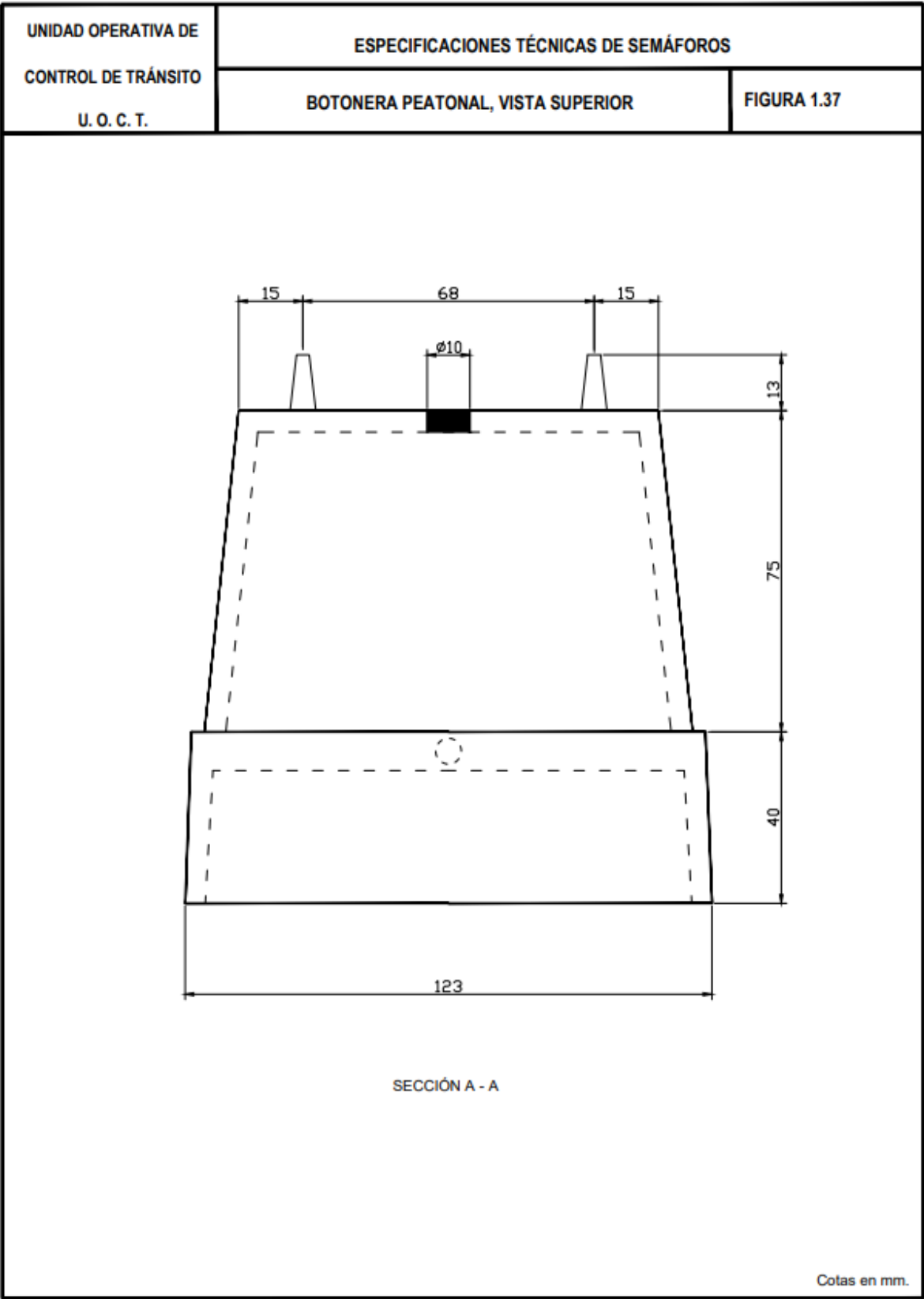
Figura 1.37 Botonera peatonal, vista superior
